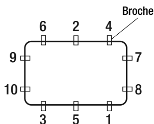
Secuencia de ajuste para las presillas
