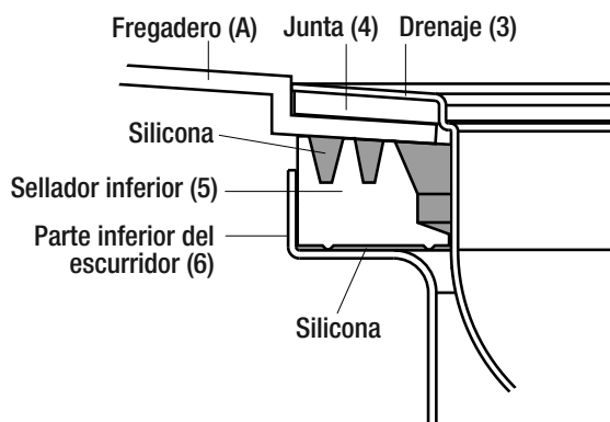
DETALLE DE LA INSTALACIÓN DEL DRENAJE
