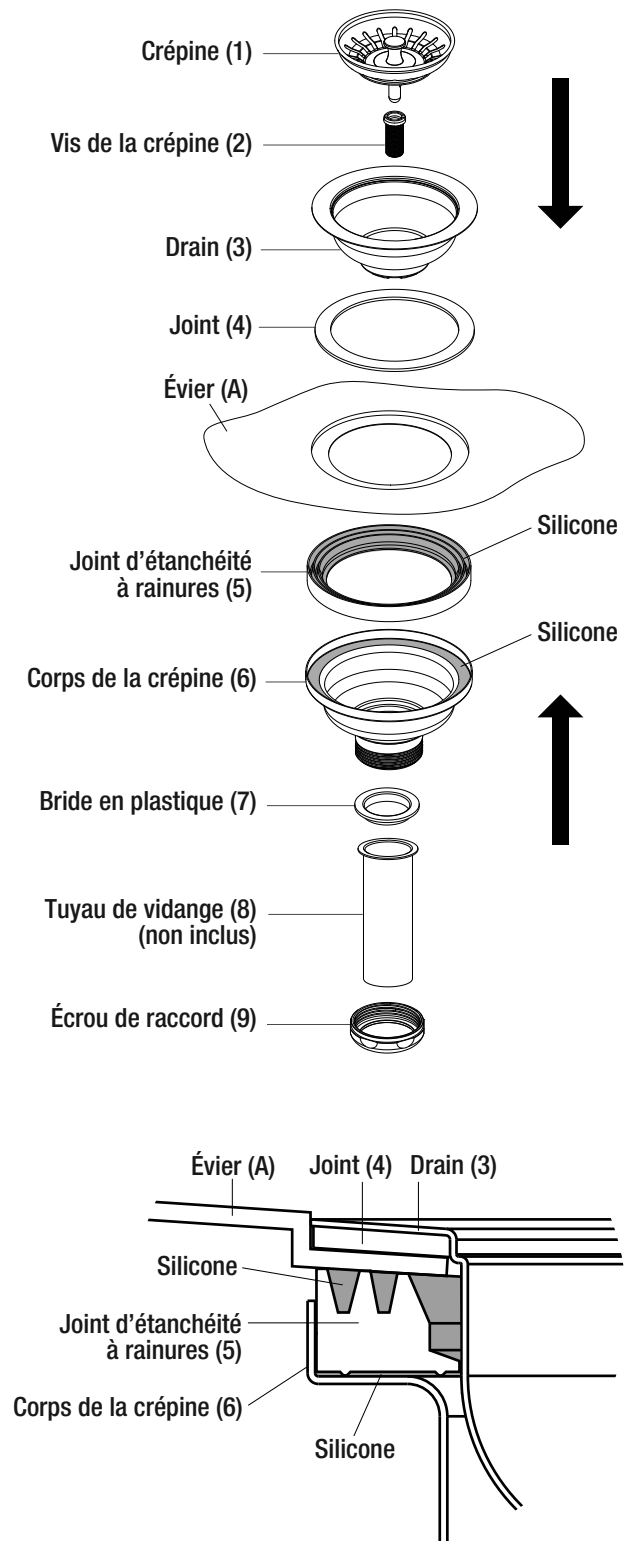
DÉTAIL DE L'INSTALLATION DU DRAIN
