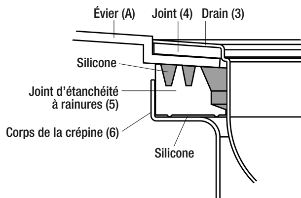
DÉTAIL DE L'INSTALLATION DU DRAIN
