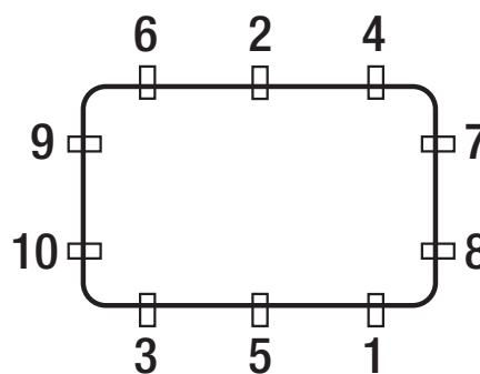
Séquence de serrage pour les attaches
