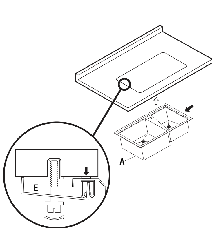
Séquence de serrage pour les attaches
