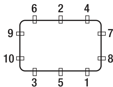
Séquence de serrage pour les attaches
